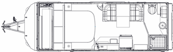
Traxx 5.9
