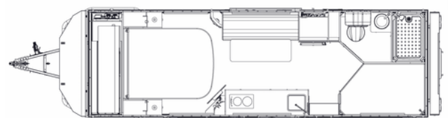
Traxx 7.2F
